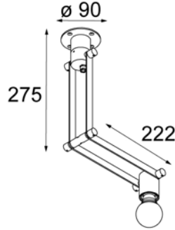
Short E27 alu
