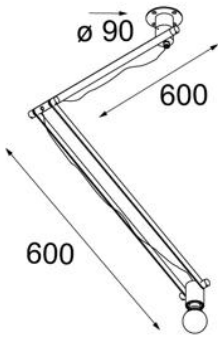
Tall E27 alu
